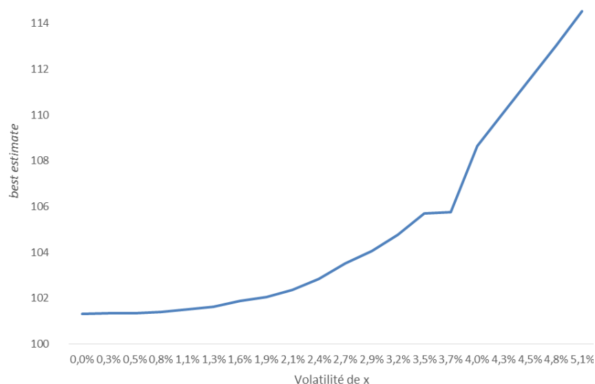
Fig. 1 : Best Estimate et volatilité du processus x
